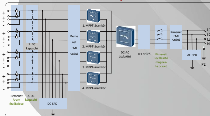
Áramköri rajz
