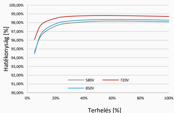
Hatásfok görbe
